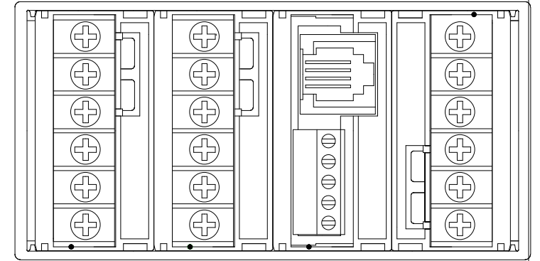
RS485ユニット RS232C+アナログ出力 RS485+アナログ出力
