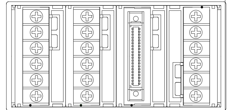
BCD出力ユニット
