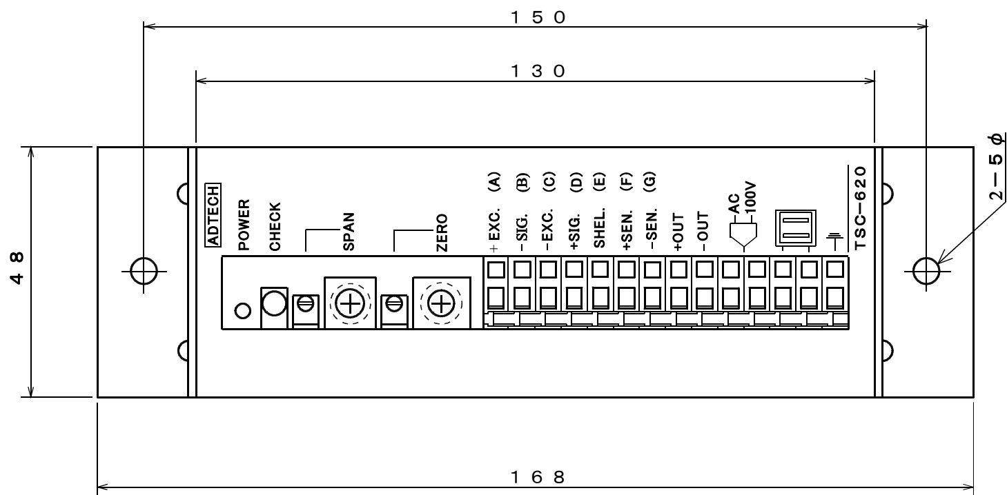
前面図
